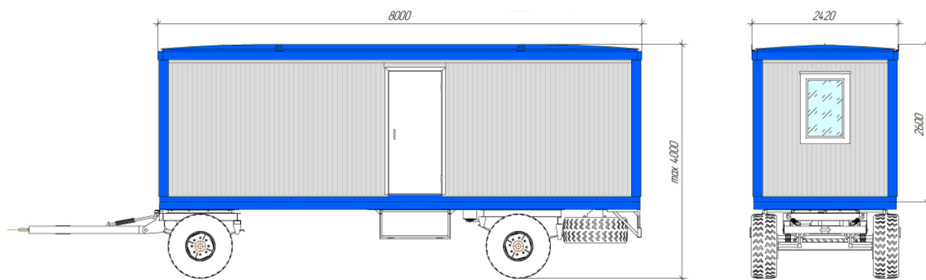
Внешний вид модульного блока на ходовой (ставни на окнах условно не показаны)
